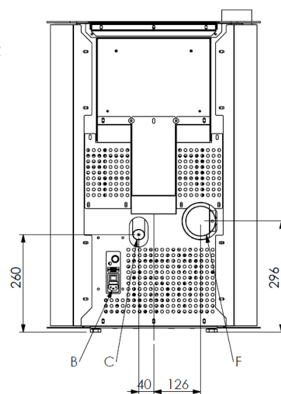
Abmessungen Pelletofen VISION ERMETICA
