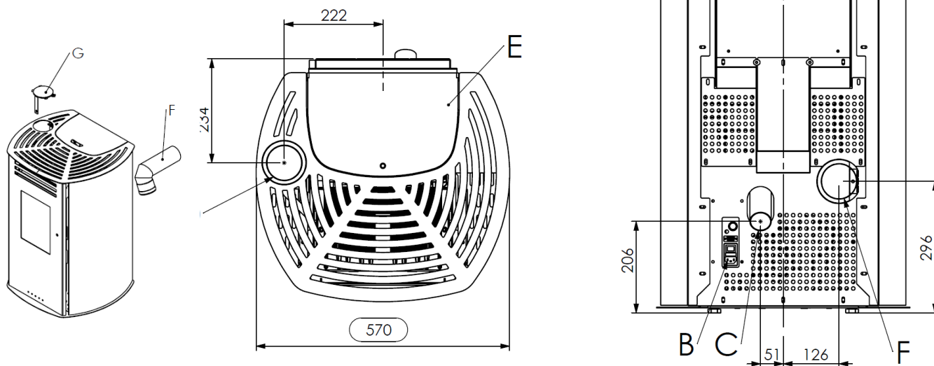
Ingombri stufa pellet VISION ERMETICA
