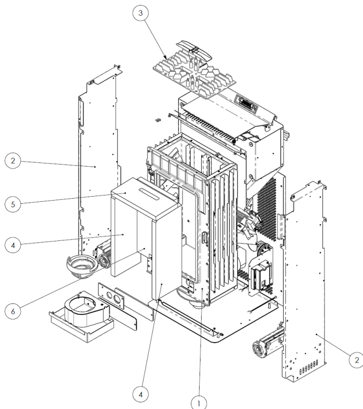
Éclaté de la chambre de combustion et des parties reliées réf. poêle VISION ERMETICA
