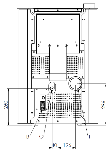
Dimensions du poêle à granulés VISION ERMETICA
