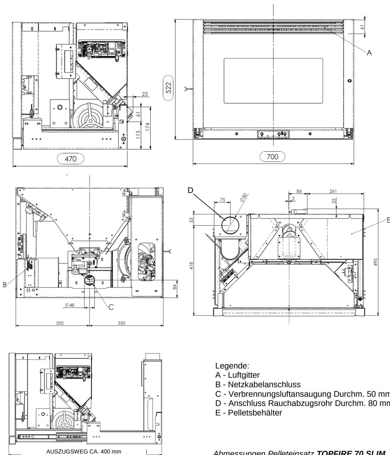
Abmessungen Pelleteinsatz TOPFIRE 70 SLIM
